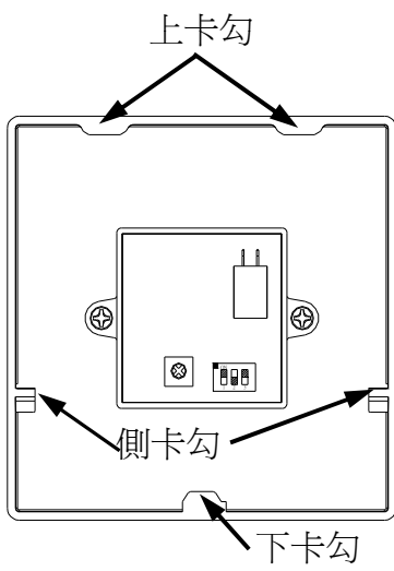
面板組背面
