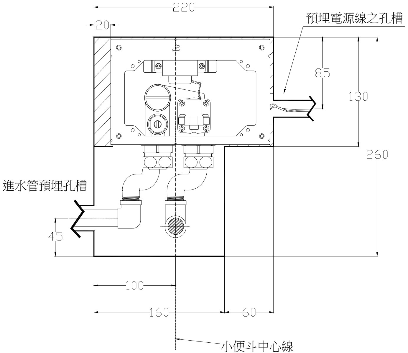
UF534(長型) 外框安裝尺寸
